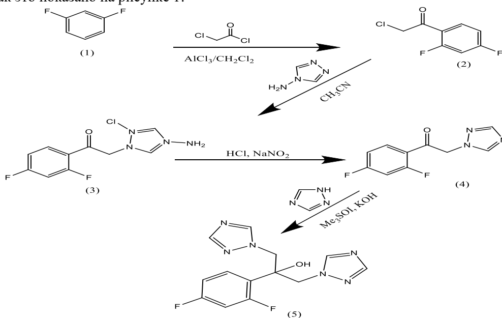
Рис. 1. Синтез Флуконазола
