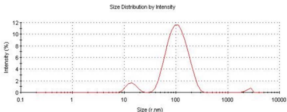
Рисунок 2. Распределение наночастиц Pd по размерам, полученных путем обработки электрическим переменным током, 50 Гц
