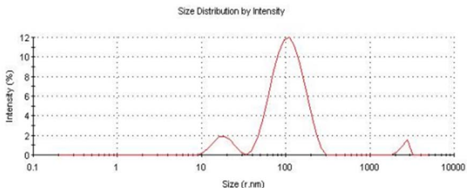
Рисунок 3. Распределение наночастиц Pd по размерам, полученных при совместном действии боргидрида натрия и электрического переменного тока, 50 Гц
