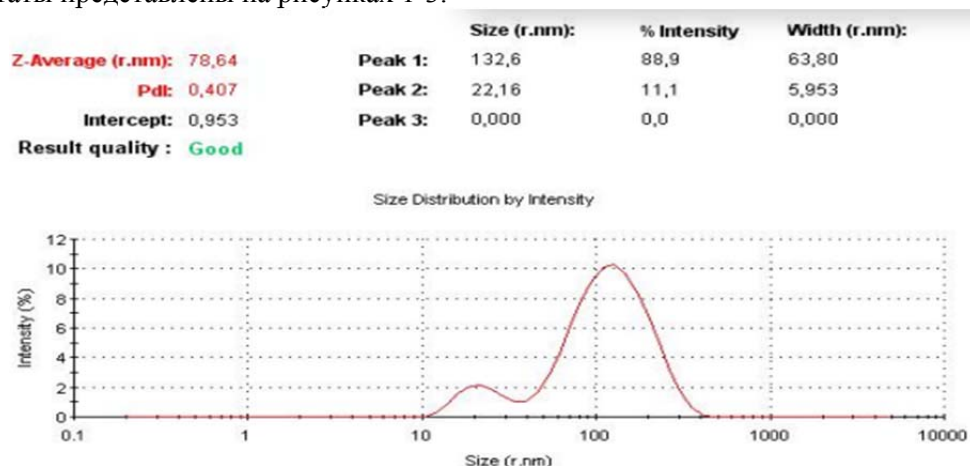
Рисунок 1. Распределение наночастиц Pd по размерам, полученным путем химического восстановления боргидридом натрия (NaBH 4 )
